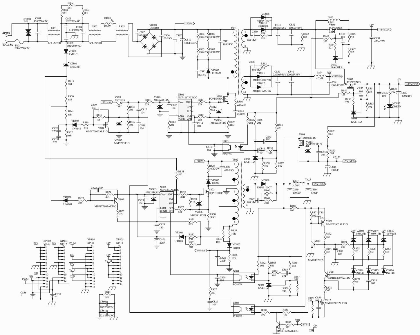
海信液晶TLM3233H 系列（1032 板）电视机电源电路原理图
